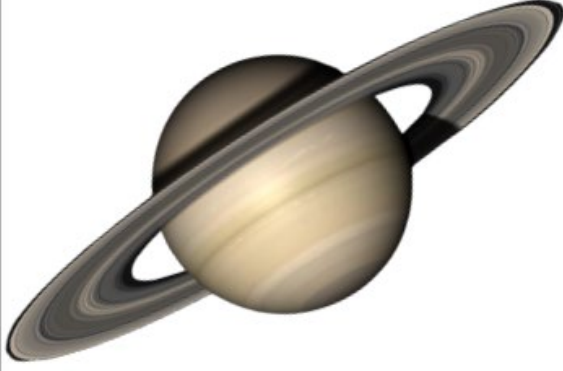
SATÜRN
