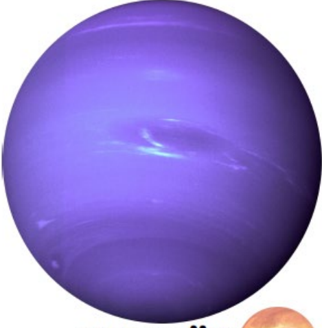
NEPTÜN
