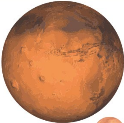
MARS fenusbilim.com
