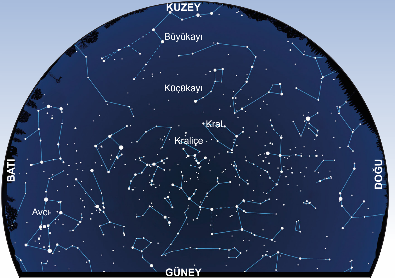
Görsel 1.2.4: Takımyıldızlar
