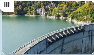
III Barajda biriken su
