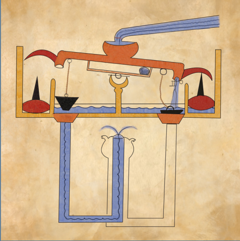
Cezerî'nin tasarladığı iki şamandıralı fiske çizimi
