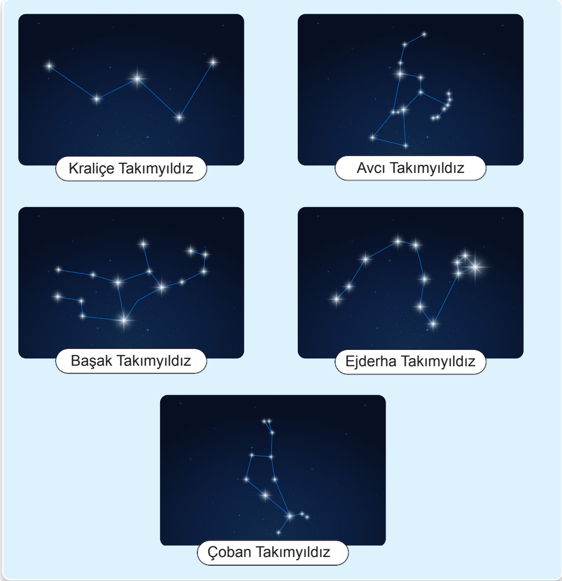
Görsel 1.2.6: En çok bilinen takımyıldızlar
