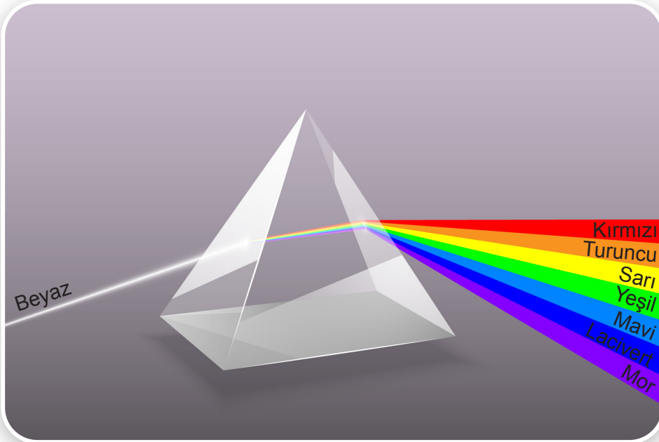
Görsel 4.1.6: Işık ışınının prizmada kırılması
