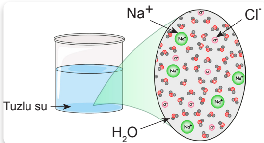
Görsel 5.3.7: Tuzun suda çözünmesi
