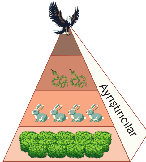
Görsel 7.1.4: Ekoloji piramidi
