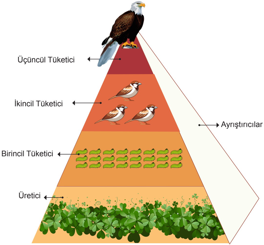
Görsel 7.1.5: Ekoloji piramidi
