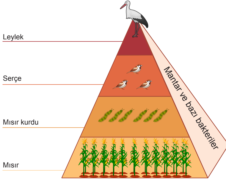
Görsel 7.1.6: Biyolojik birikim ve ekoloji piramidi
